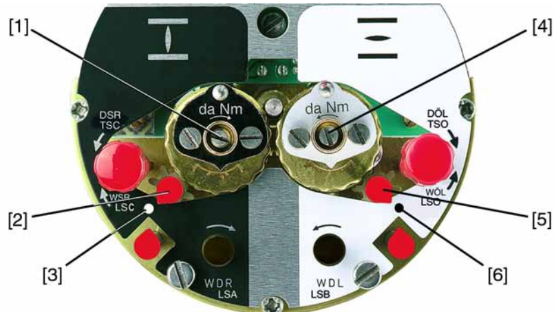
рис. 23: Регулировочные элементы концевого выключателя
